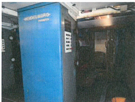
Foto 1, Linea per stampa rotativa 32 pagine
