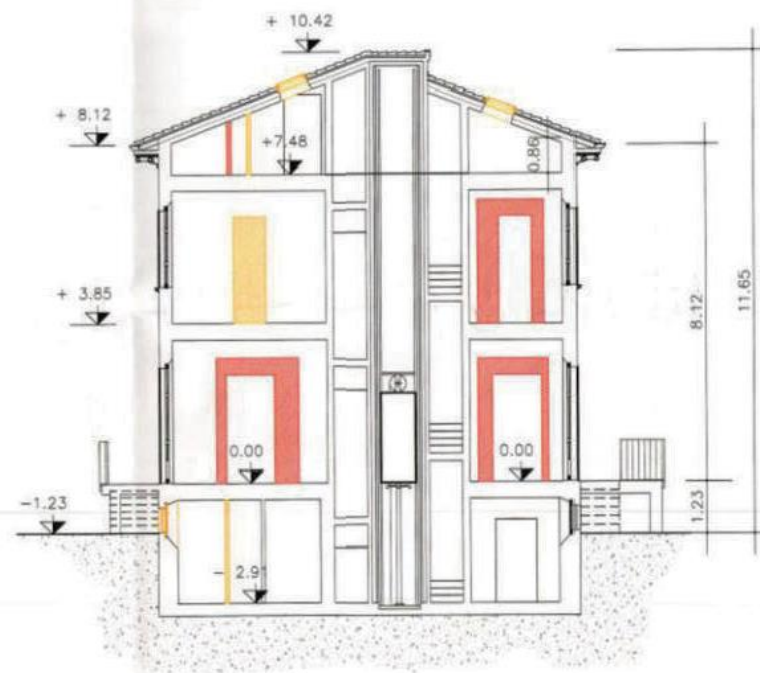
SEZIONE B-B'
