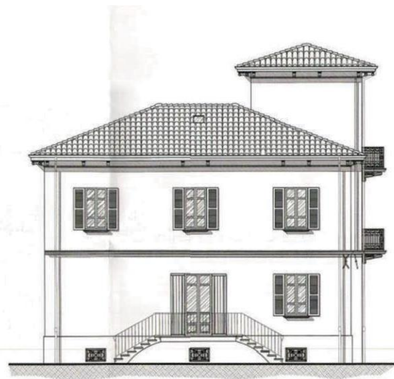
PROSPETTO SUD-OVEST
