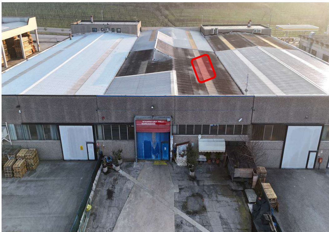
*FOTO AEREA DELLA COPERTURA CON DRONE- NEL RIQUADRO ROSSO LA ZONA DI INFILTRAZIONE RISCONTRATA NEL CORSO DEL SOPRALLUOGO
