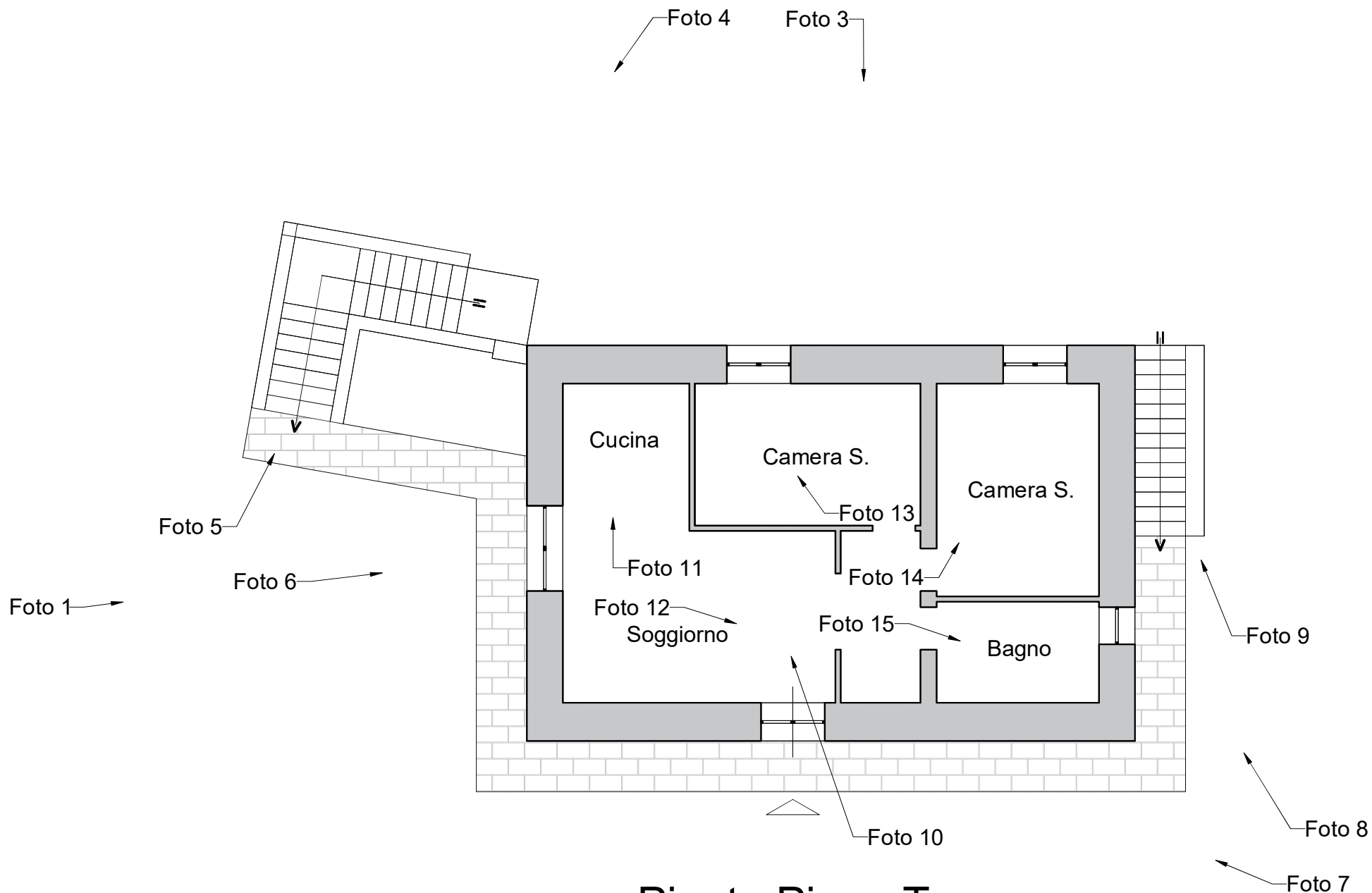
Pianta Piano Terra Riferimenti fotografici
