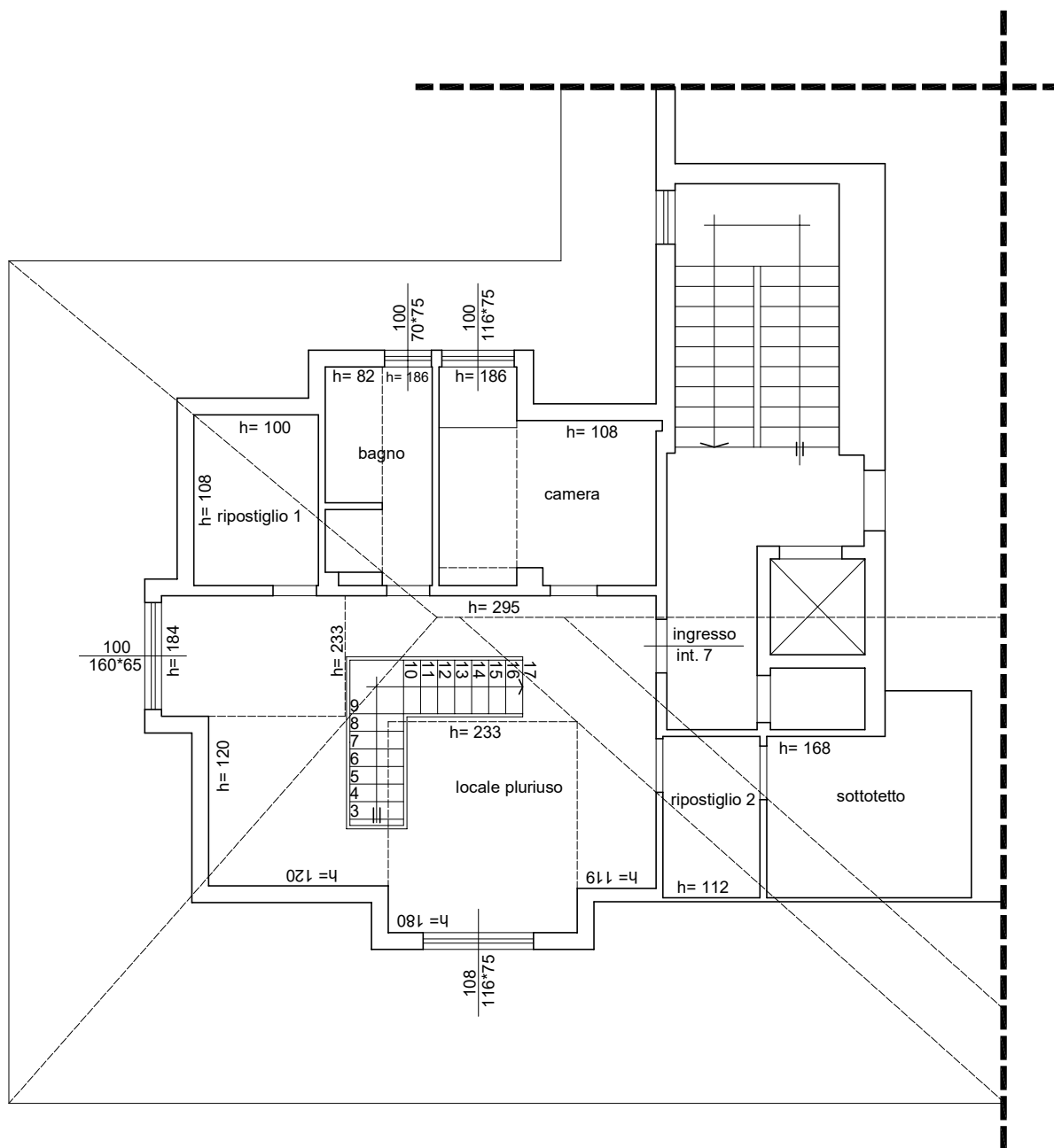
PIANO QUARTO/SOTTOTETTO (STATO DI FATTO) RAPP. 1:100
