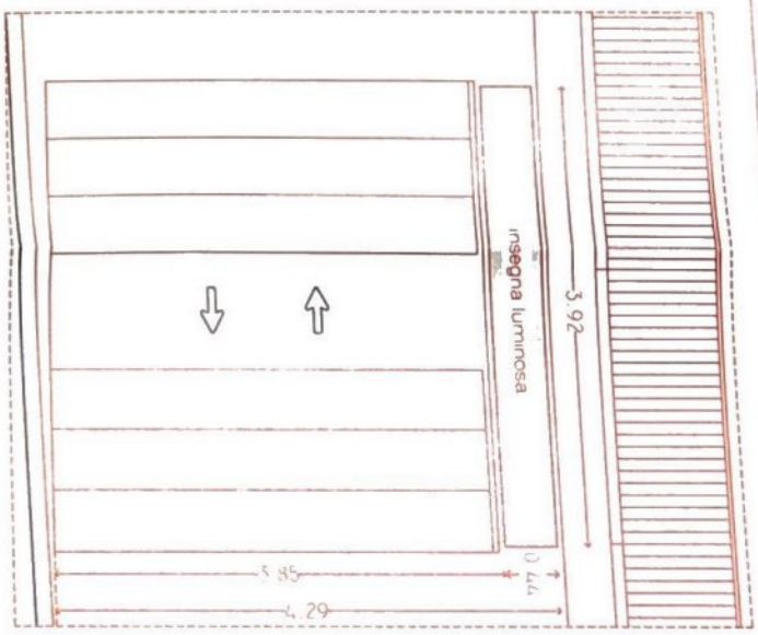
PROSPETTO OVEST situazione di progetto
