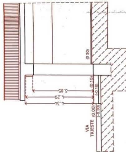
SEZIONE di fatto
