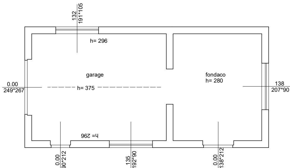
PIANTA PIANO TERRA IMMOBILE "A" RAPP. 1:100
