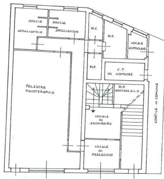
PIANTA PIANO TERRA H = 3.37
