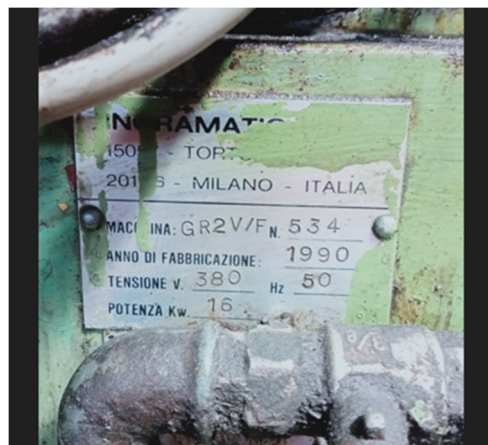
Figura 30 Targhetta.
