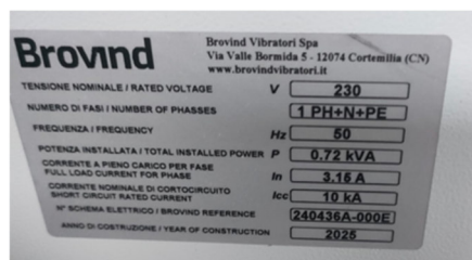
Figura 5 Targhette caricatore.
