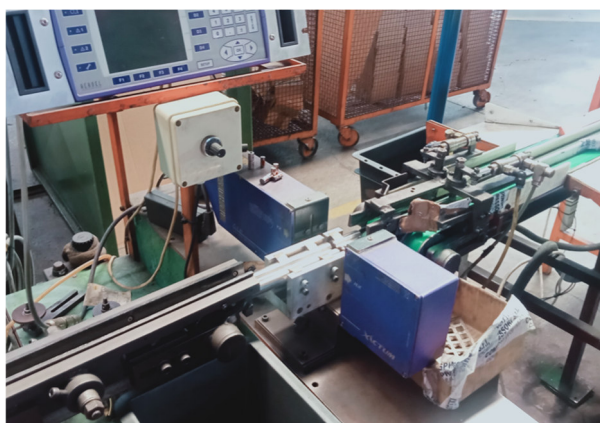
Figura 23 Sistema laser di controllo dimensionale.
