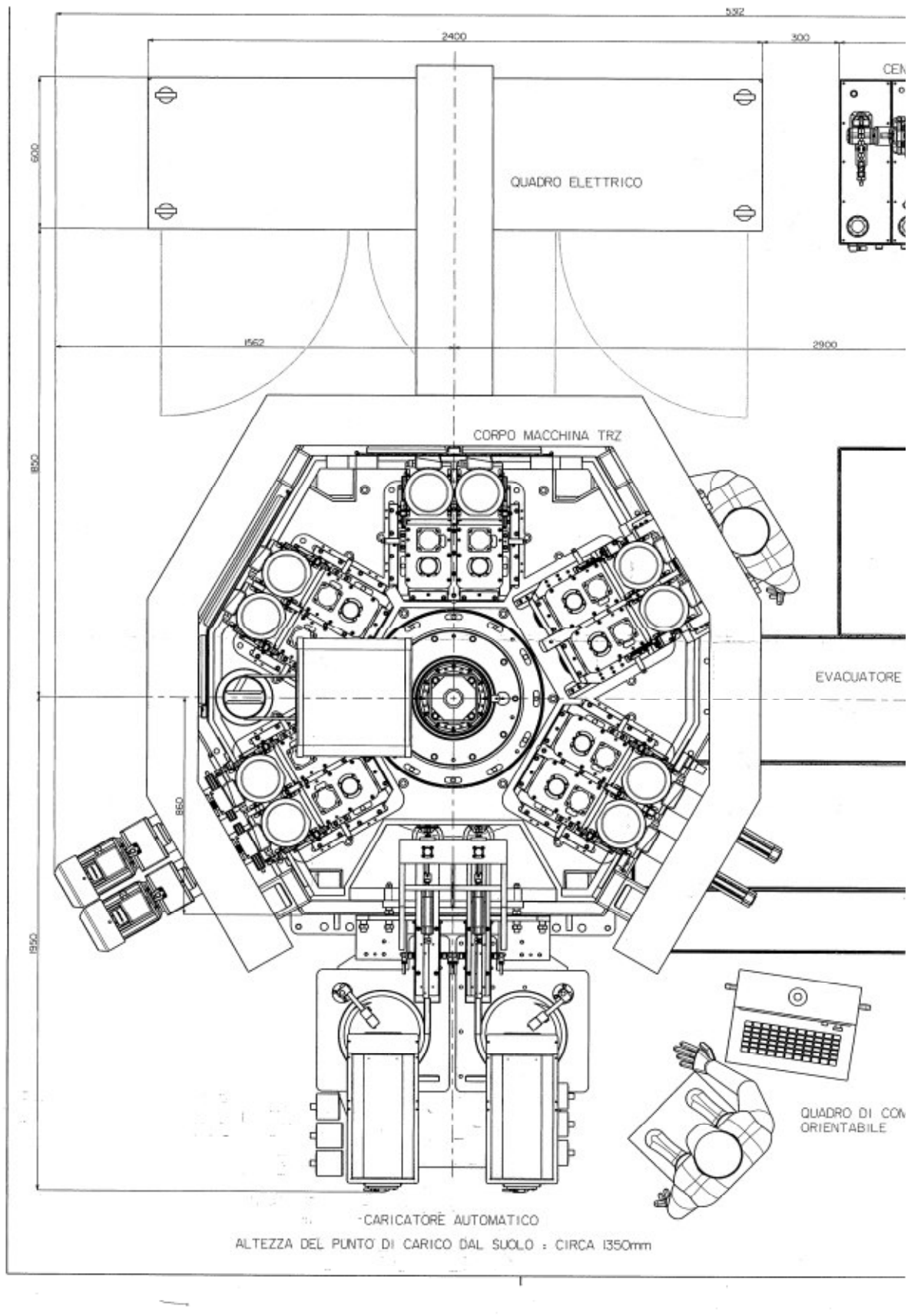
Figura 2 Lay-out generale della linea TRZ
