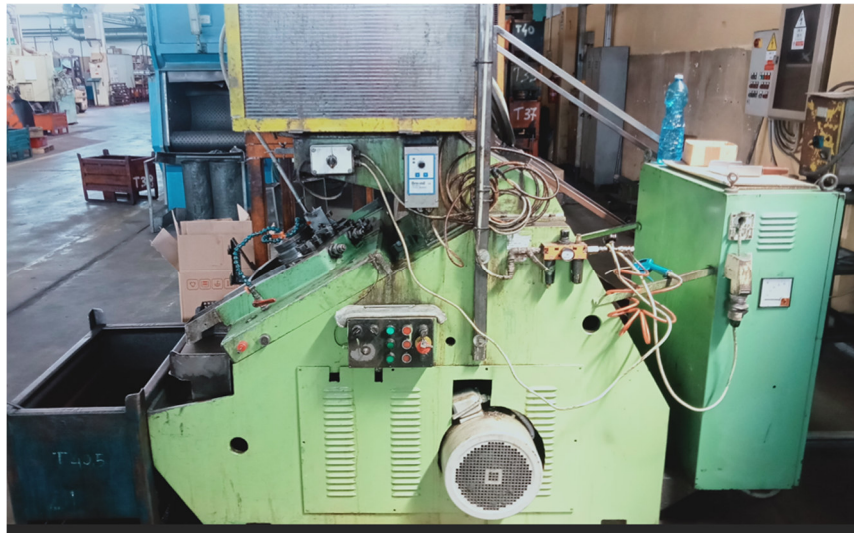
Figura 29 Rullatrice Ingramatic.
