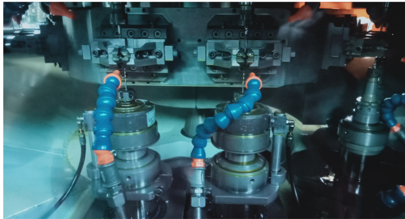
Figura 7 Dettaglio interno macchina.
