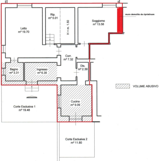
Planimetria dell'int. 1, posto al p t – 1° lotto
