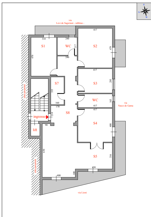
Fig. 1.d –rilievo dello stato di fatto dell'immobile inserito nel NCEU al fg. 111 p.lla 986 sub 6
