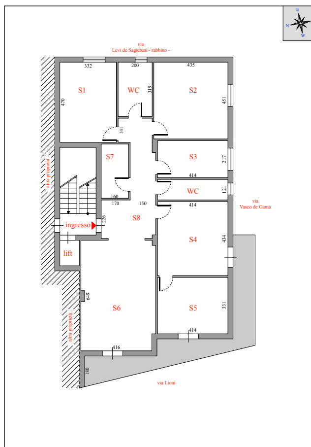
Fig. 1.a –rilievo dello stato di fatto dell'immobile inserito nel NCEU al fg. 111 p.la 986 sub 3
