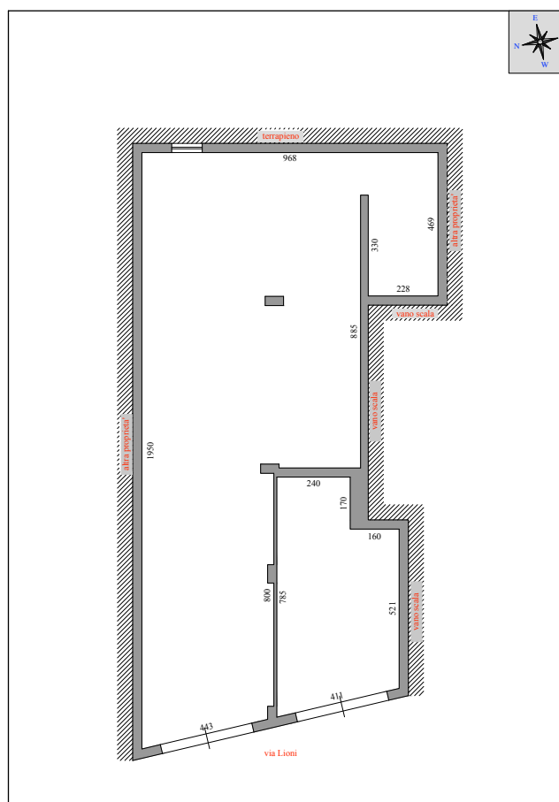
Fig. 1.f –rilievo dello stato di fatto dell'immobile inserito nel NCEU al fg. 111 p.la 986 sub 12
