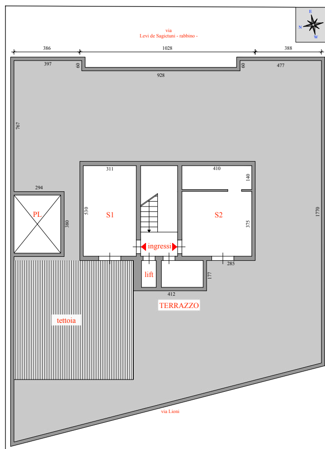
Fig. 1.c –rilievo dello stato di fatto dell'immobile inserito nel NCEU al fg. 111 p.la 986 sub 10
