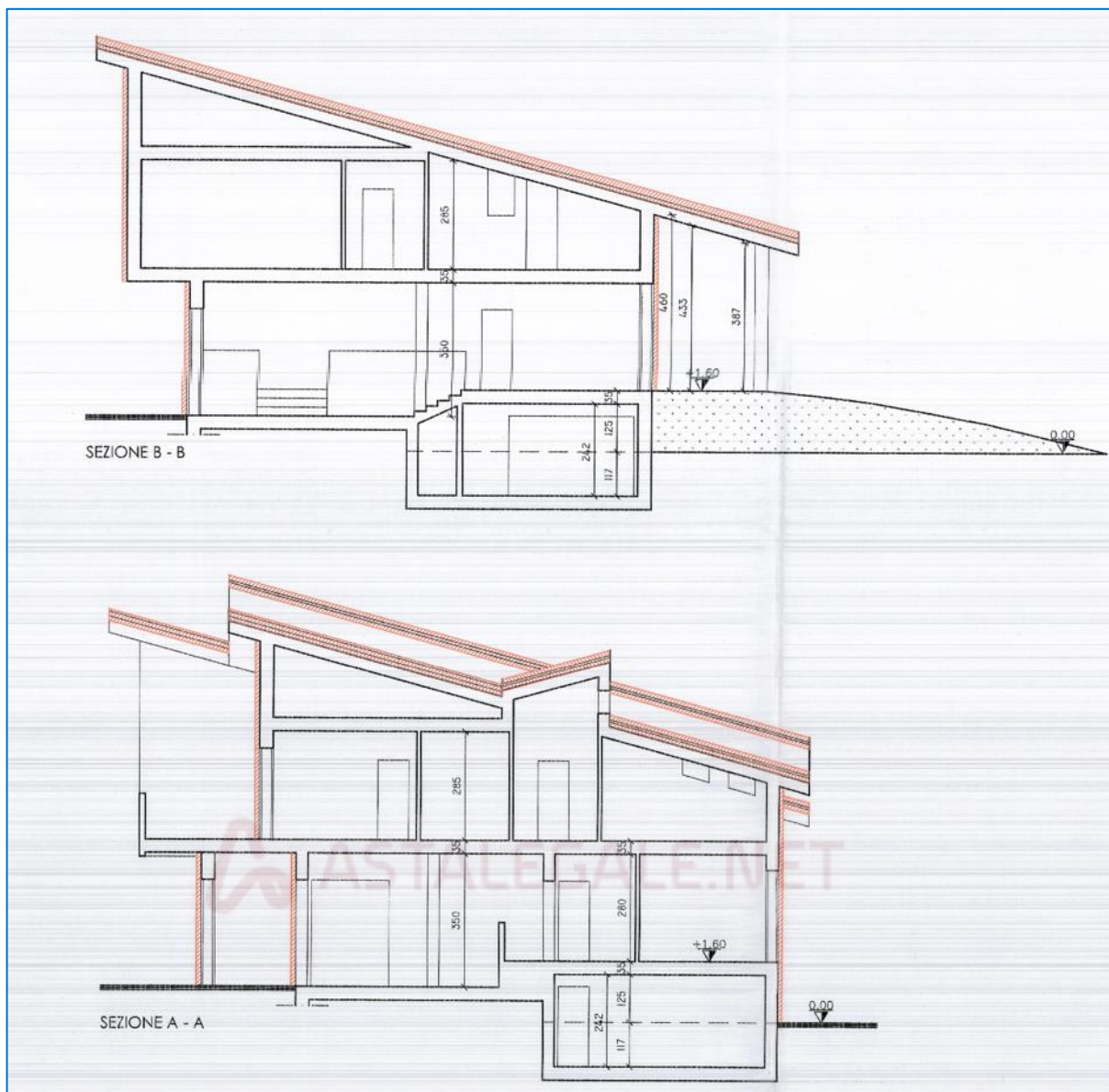
5. Sezioni.
