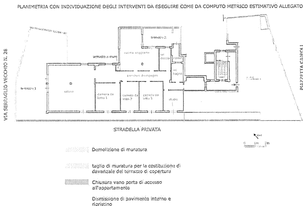
Grafici dei lavori descritti nel computo metrico estimativo (All. 33a)
