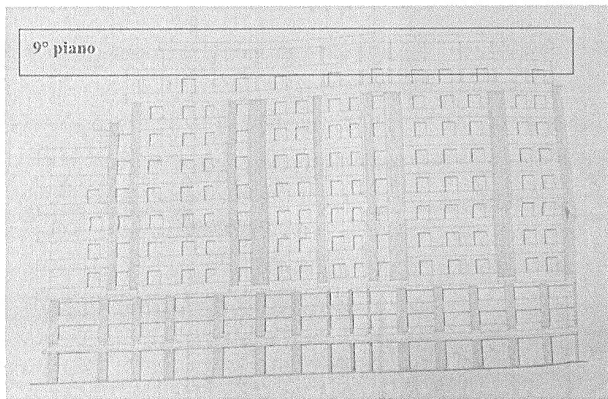
Estratto grafico del Progetto di variante di cui alla C.E. del 13.11.1972 variante n. 549 del 20.06.1973 Prospetto su stradella privata (All. 16)
