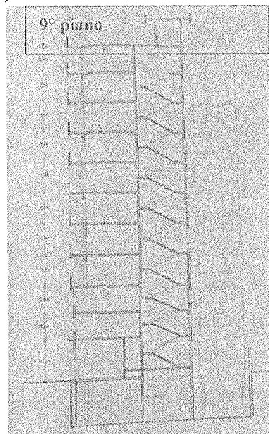
Estratto grafico del Progetto di variante di cui alla C.E. del 13.11.1972 variante n. 549 del 20.06.1973 Prospetto su via Serraglio Vecchio n. 28 e sezione trasversale (All. 16)
