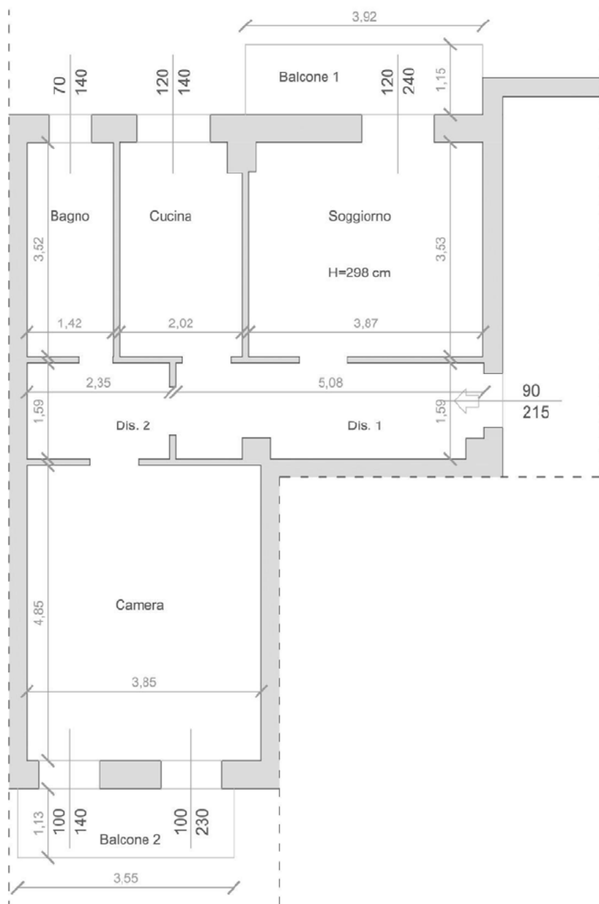
Fot. 1 - Pianta appartamento
